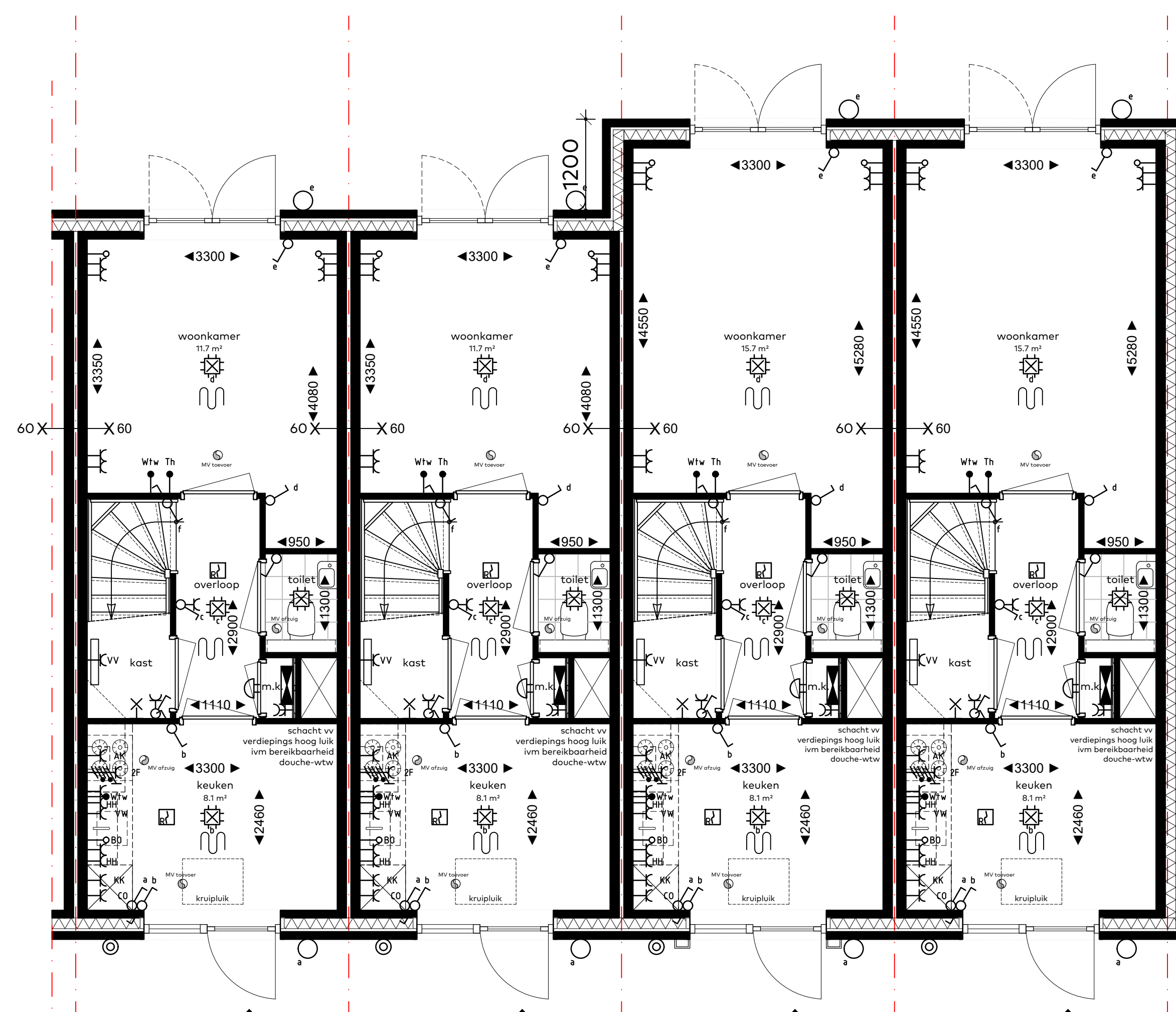
Begane grond Woningen (blok 3)
