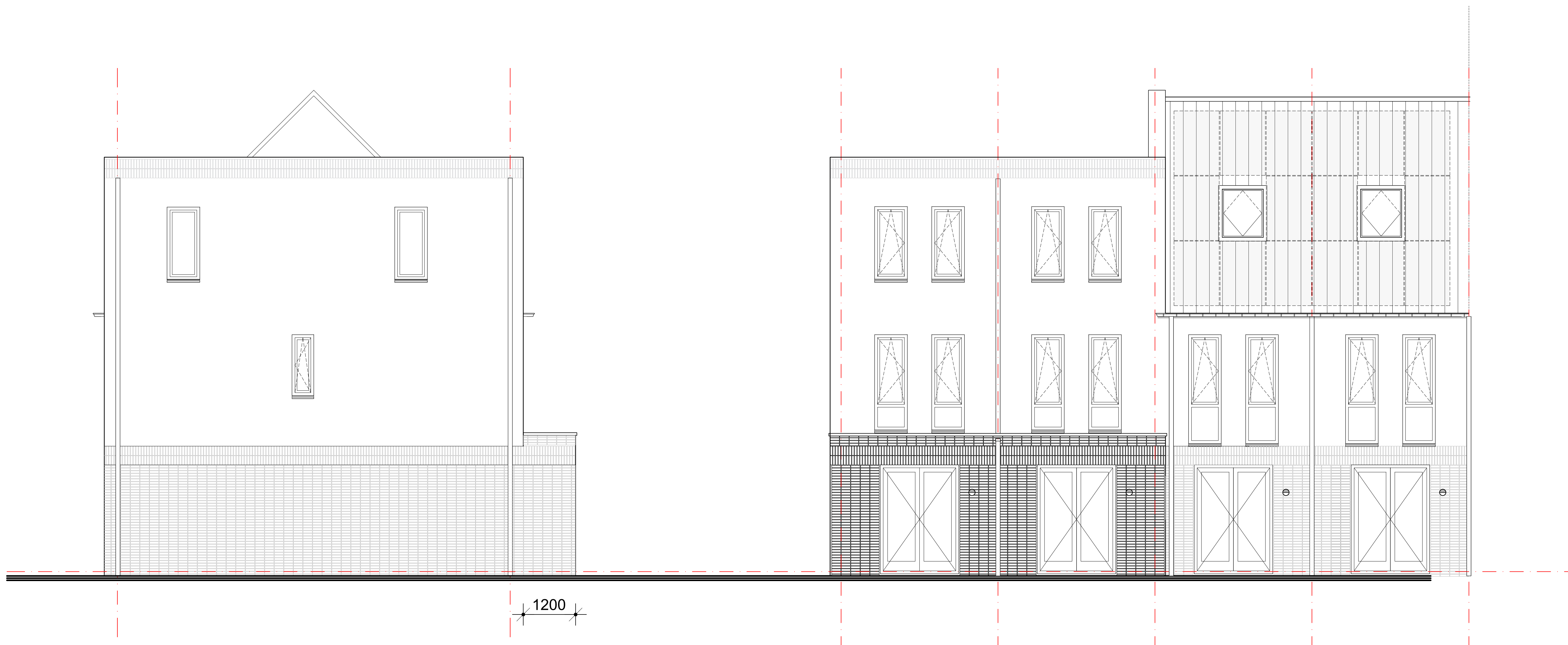
Zijgevel 3,6m woningen (blok 3)
