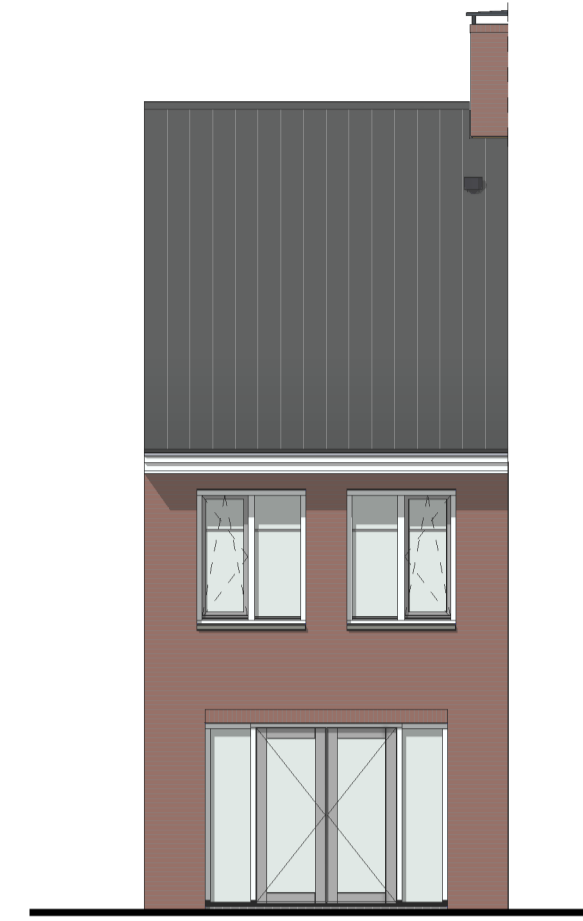
Achtergevel
