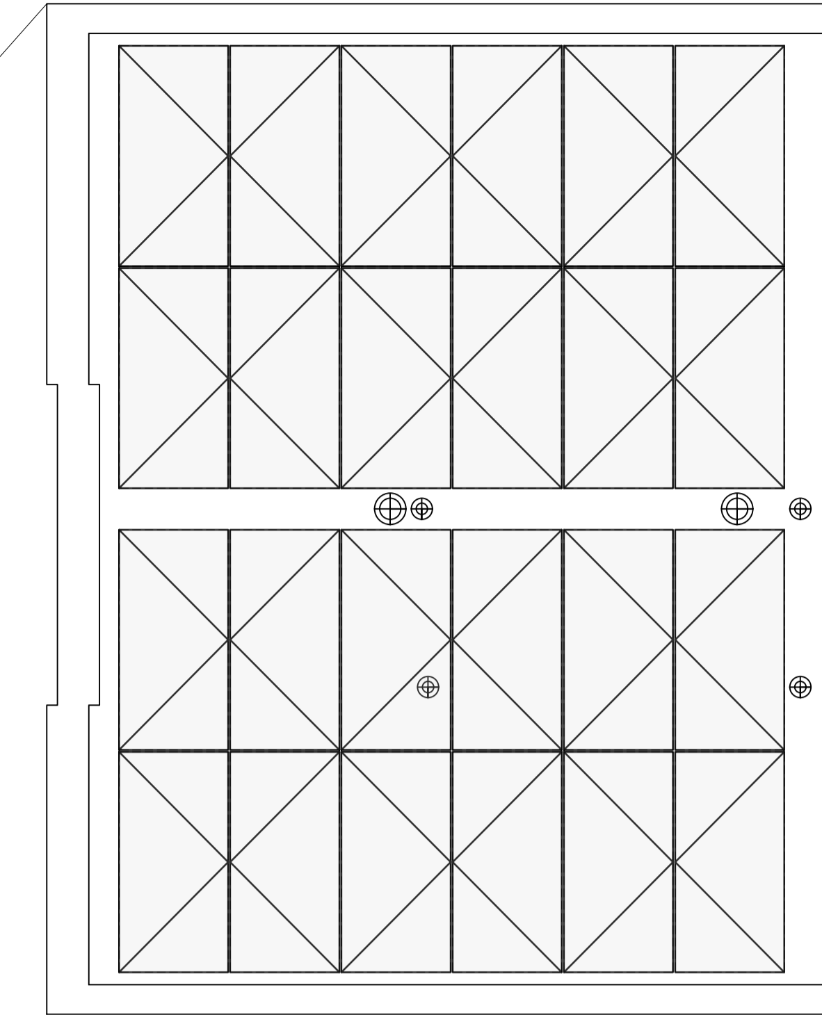
PV-panelen volgens E-installatie tek. (aantal en exacte positie conform BENG-berekening) plattendak
