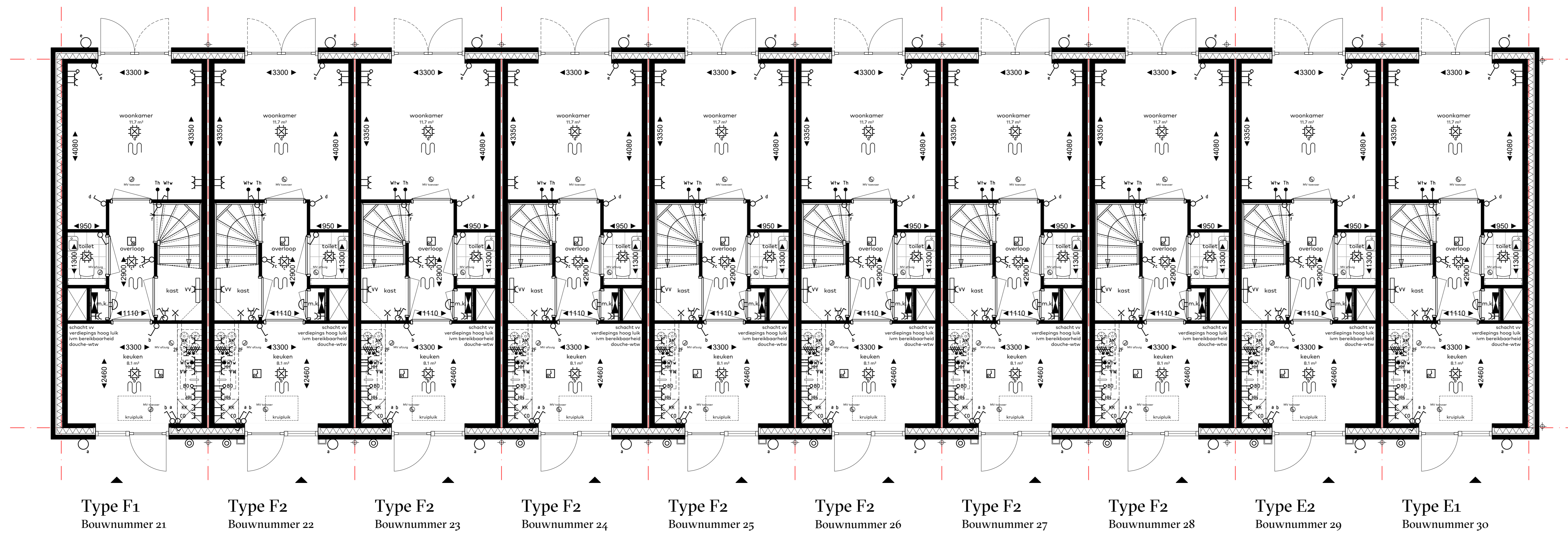
Begane grond, blok 3
