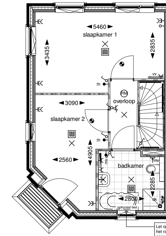
Eerste verdieping
