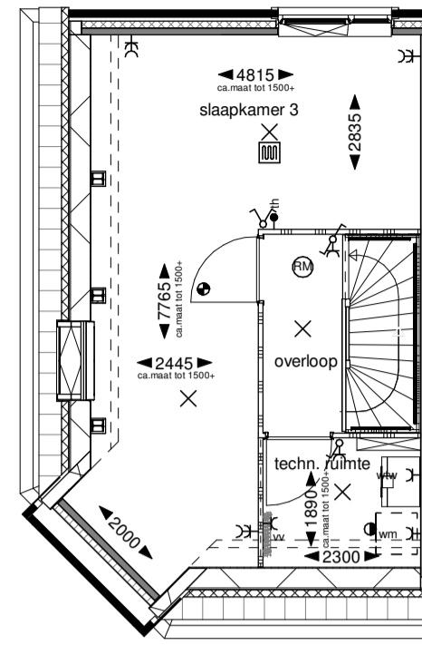
Tweede verdieping
