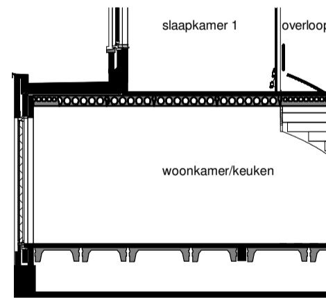
Doorsnede
