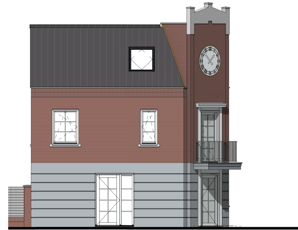
Linker zijgevel
