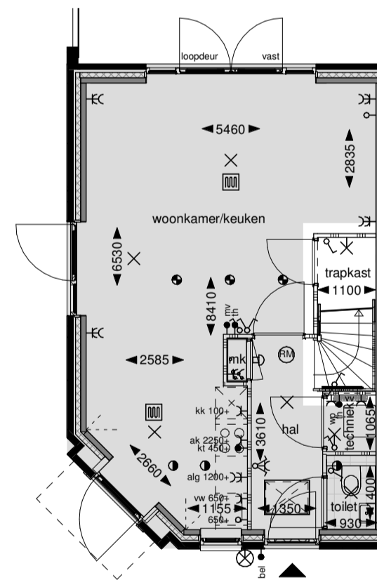
Begane grond
