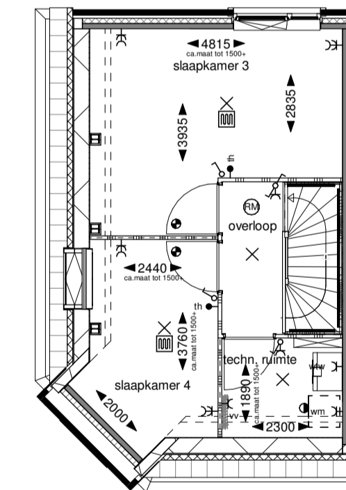
Tweede verdieping
