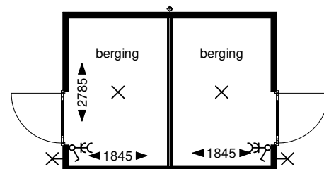
Begane grond
