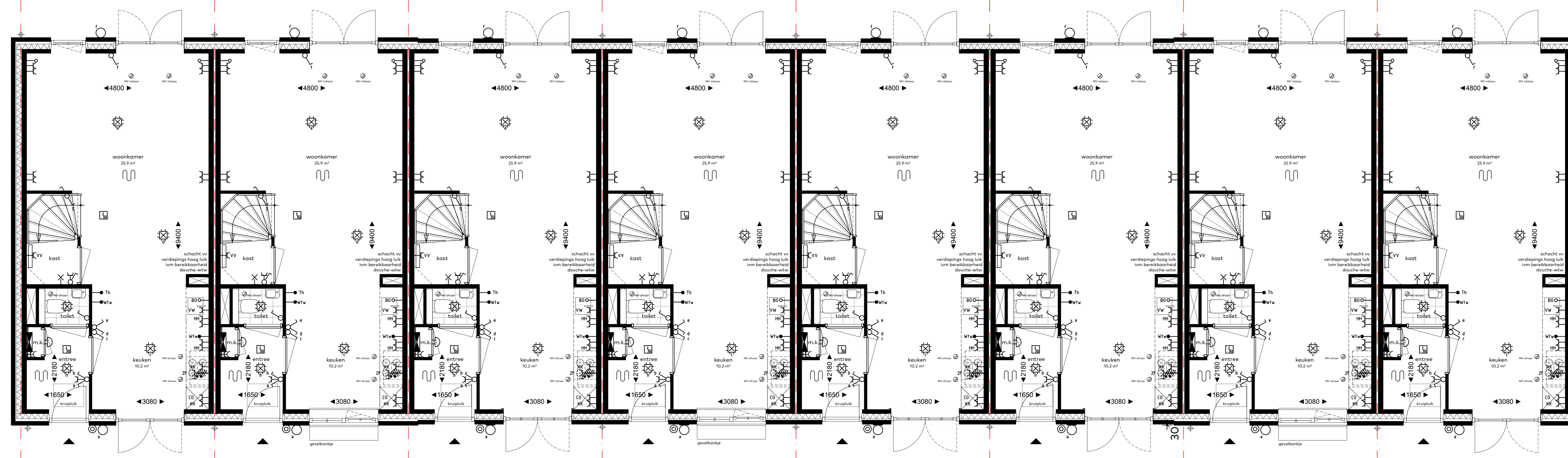
Type A4 Bouwnummer 40 Type A5 Bouwnummer 41 Type B2 Bouwnummer 42 Type B3 Bouwnummer 43 Type B2 Bouwnummer 44 Type B1 Bouwnummer 45 Type A2 Bouwnummer 46 Type A6 Bouwnummer 47 Begane grond, blok 5
