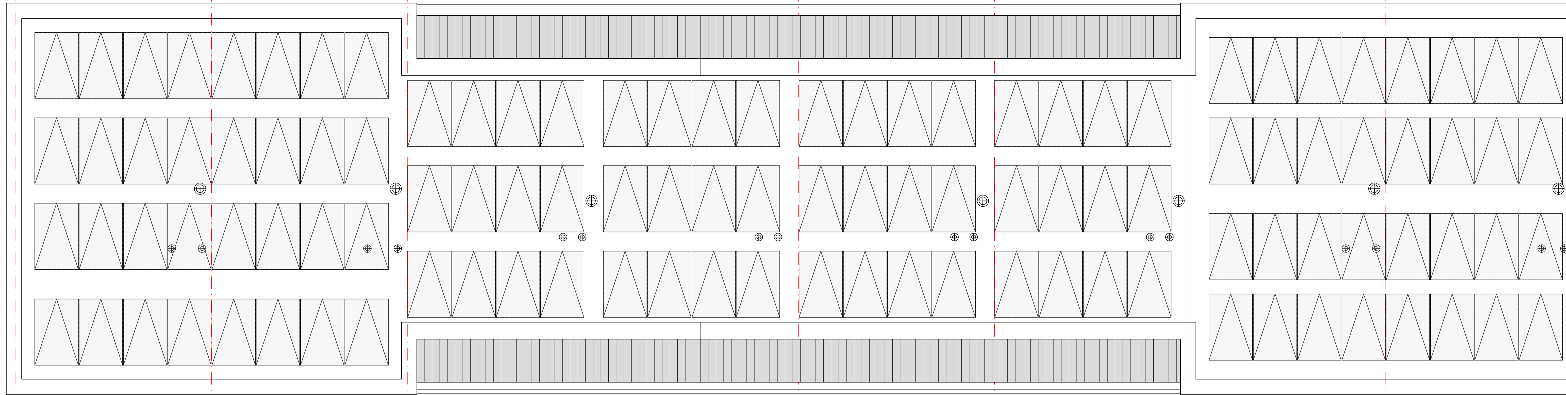
Platdak PV-panelen volgens E-installatie tek. (aantal en exacte positie conform BENG-berekening)
