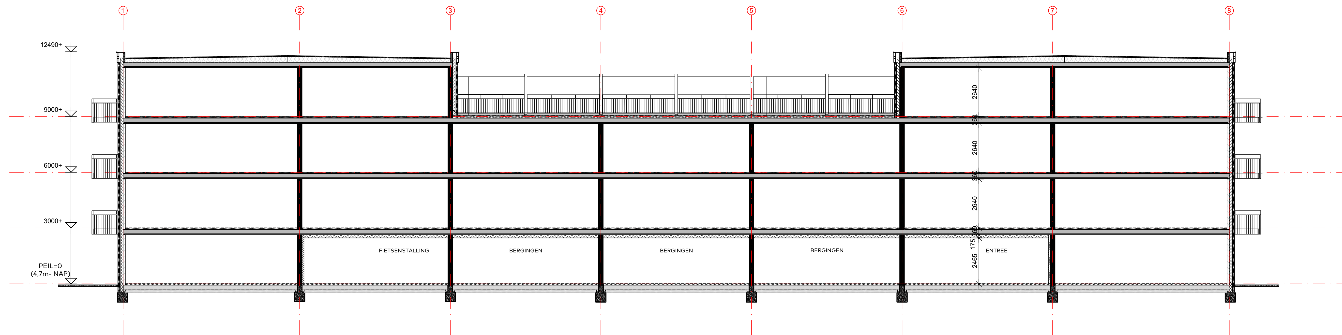
Langsdoorsnede
