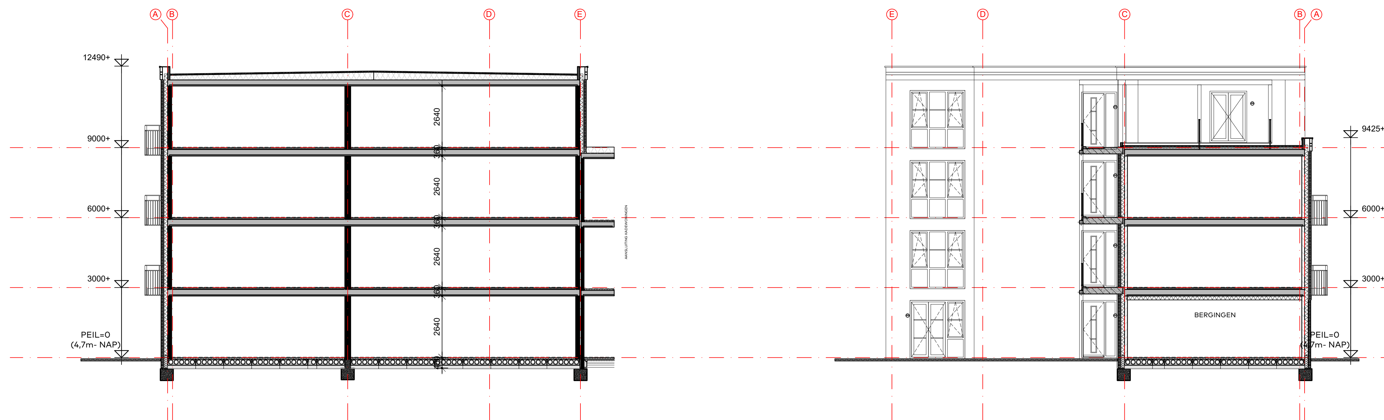
Dwarsdoorsnede A
