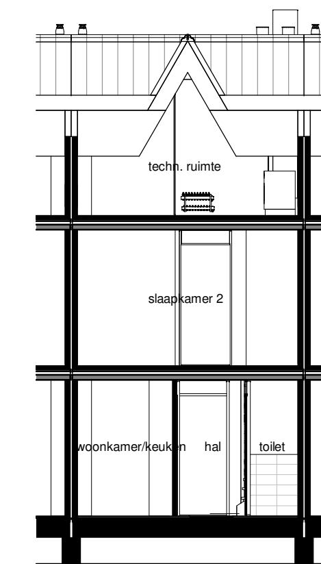
Doorsnede E-E
